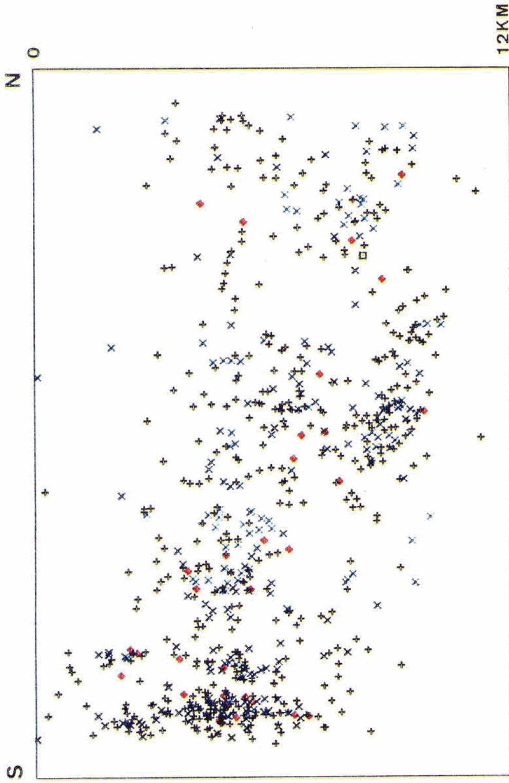
Figure V.9: Coupe de la sismicité de la faille de Calaveras, de 1969 à 1981. Croix noires = magnitude 1,5 à 2,5; x bleus = magnitude 2,5 à 3,5; losanges rouges = magnitude 3,5 à 4,5; carré vert = magnitude supérieure à 4,5.
