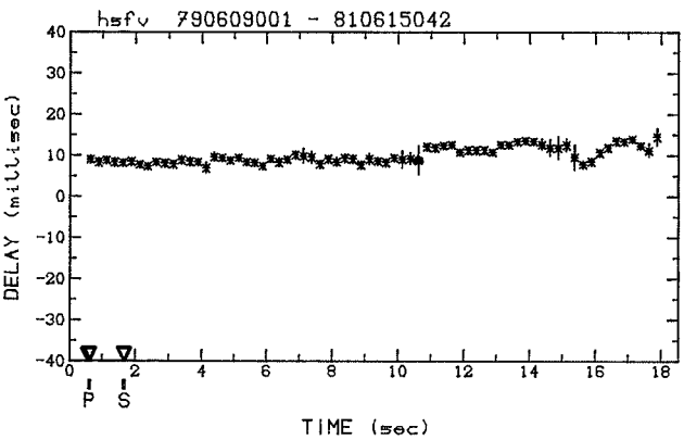
DOUBLET S4 (début)
