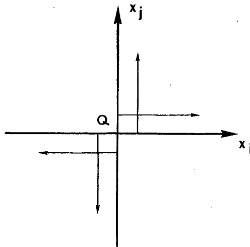
Figure 1 : Double couple M_{ij}
