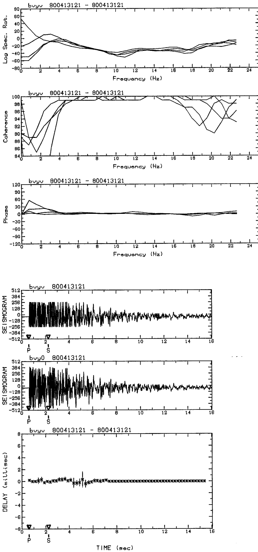
Figure 7 (suite): Idem. Ecrêtage égal à 2/3.
