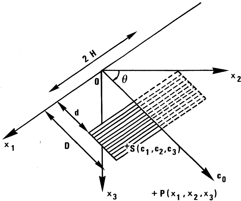
Figure 4 : Géométrie de la faille
