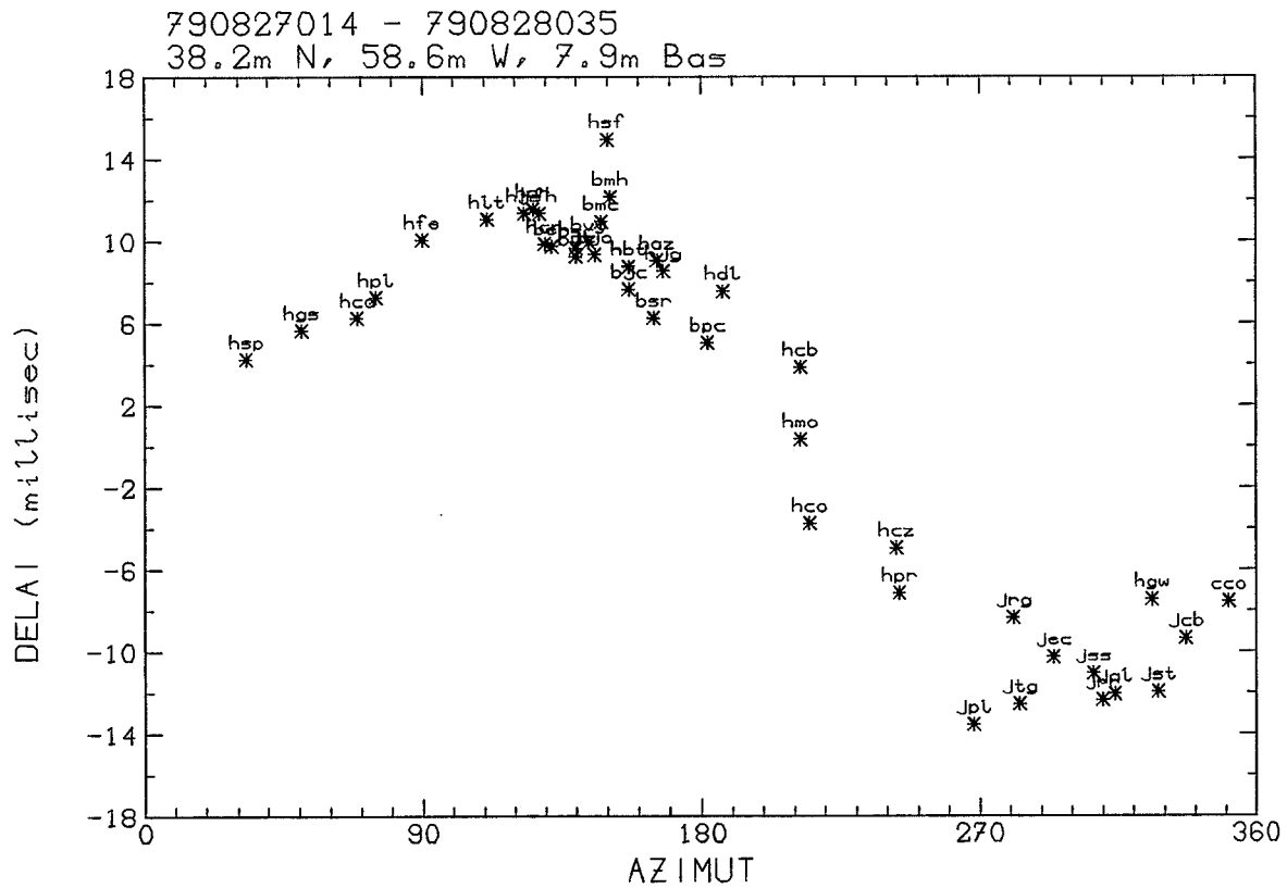
Figure V.1: Délai de l'onde P en fonction de l'azimut de la station.
