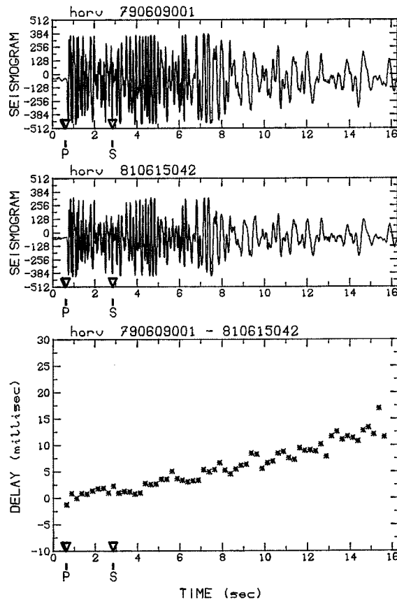
Figure 1 : Exemple de croissance linéaire du délai le long du sismogramme indiquant une diminution de vitesse de 0,08%. Le séisme de 1981 est étiré par rapport à celui de 1979 (en haut sur la figure).
