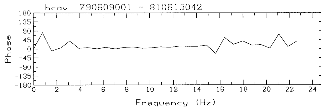
Figure 3.b : Analyse spectrale des signaux représentés Figure 3.a. On a tracé la phase de l'inter-spectre (en degrés), la cohérence (en pourcentage), le logarithme du rapport spectral ( \times 100 ), et le module de l'inter-spectre (en pourcentage du maximum). Les spectres sont non lissés.
