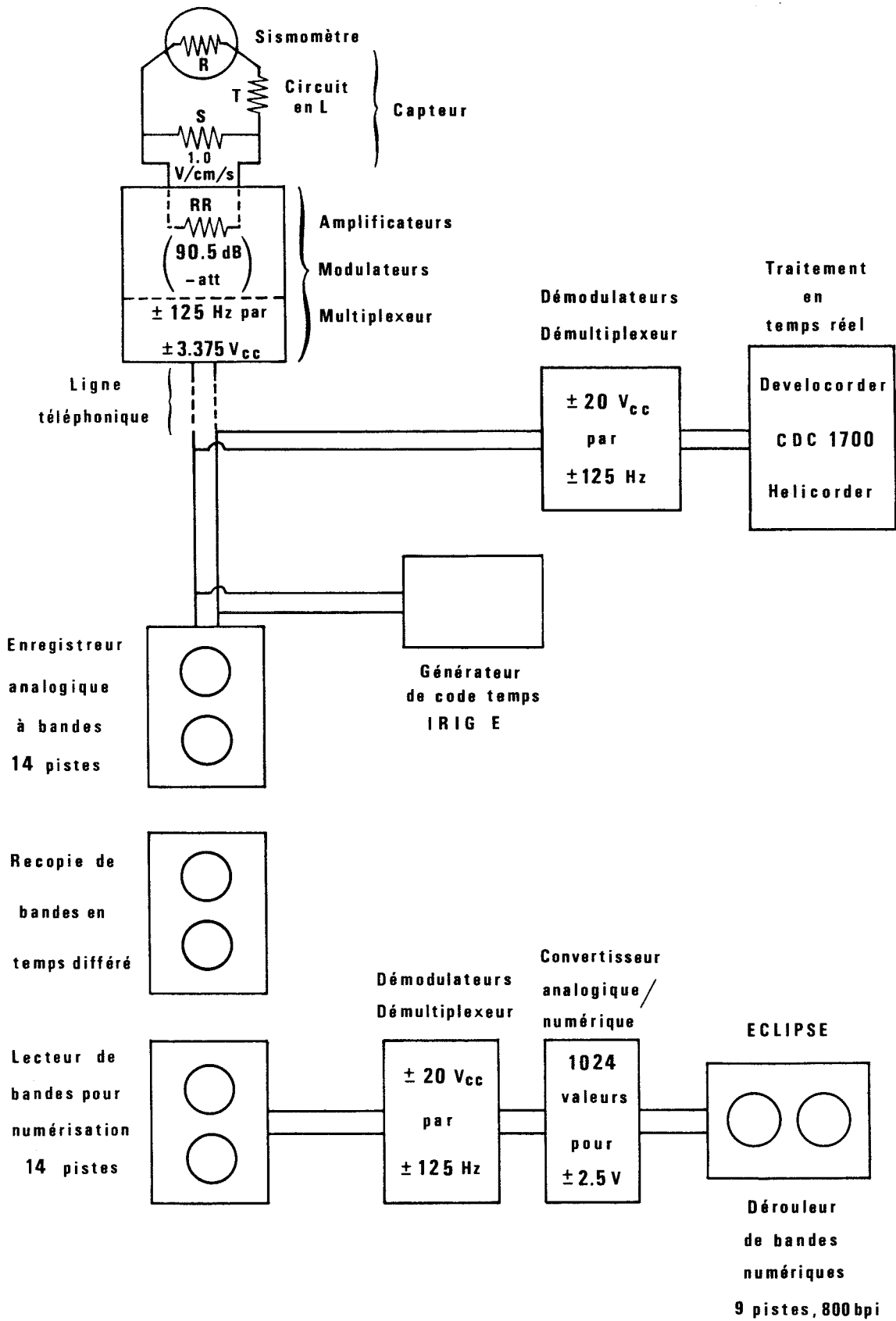
Figure IV.2: Chaîne d'acquisition des sismogrammes à l'U.S.G.S..
