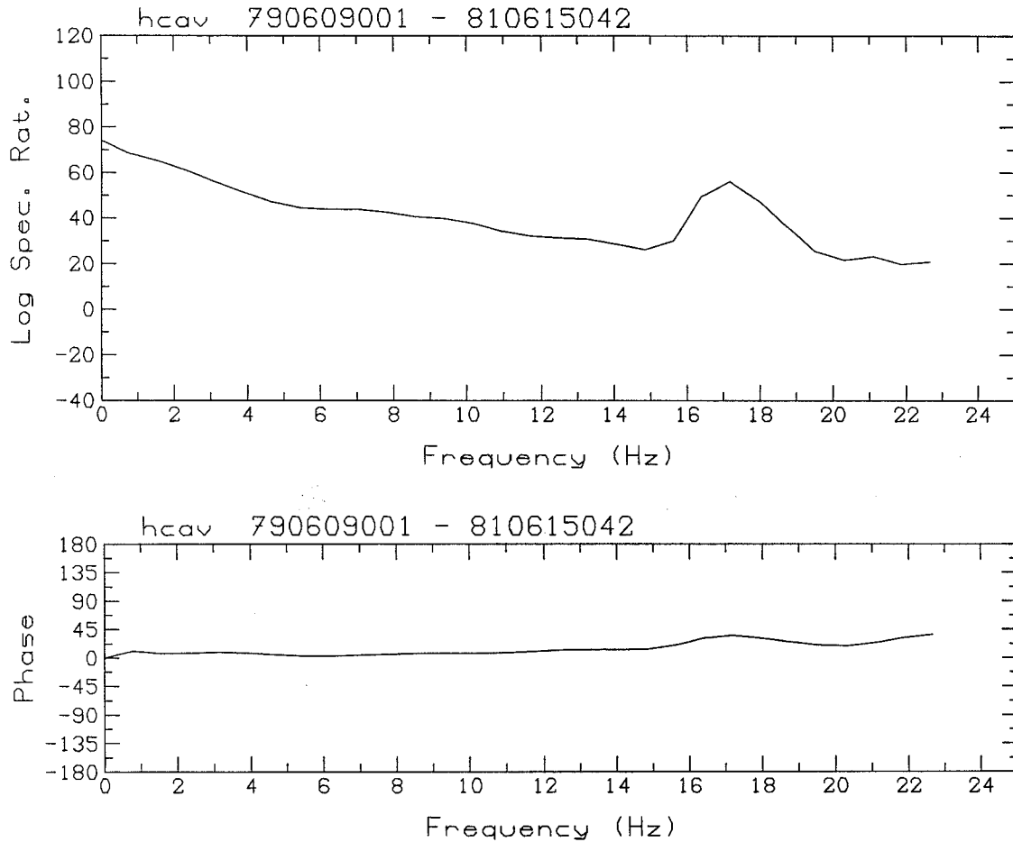
Figure 4 : Phase et rapport spectral lissés pour les signaux étudiés Figure 3.
