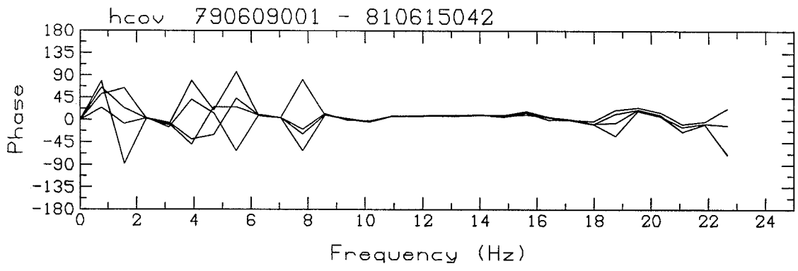
Figure 6 : Analyse spectrale d'un doublet pour des fenêtres de longueur 1.28s, déplacées successivement de 0.04, 0.08 et 0.12s. On constate le bon accord entre cohérence temporelle et cohérence fréquentielle.
