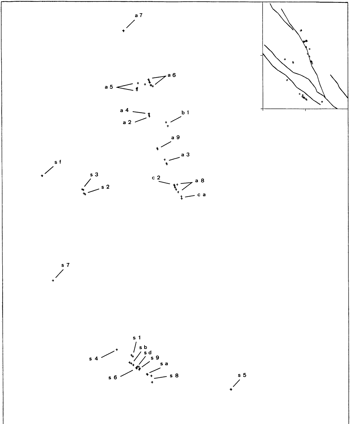
Figure V.5: Carte de l'ensemble des séismes étudiés. Les noms des doublets et des multiplets sont indiqués. En encart, position des doublets par rapport aux failles.
